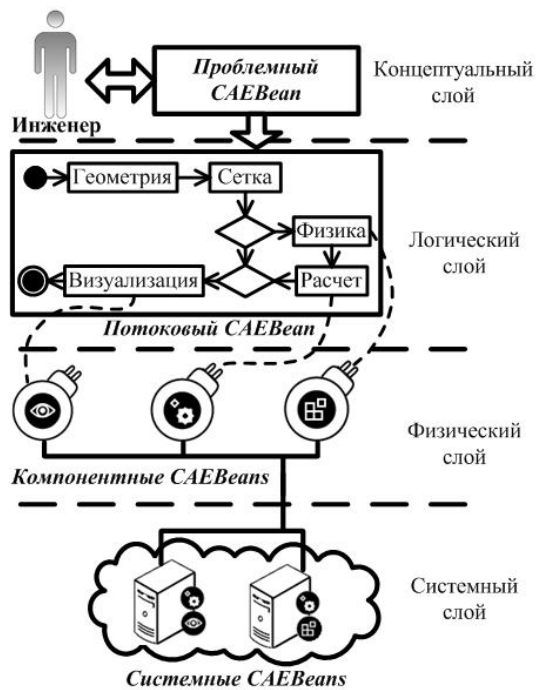
Рис. 1. Обобщенная схема слоев PaVIS.
