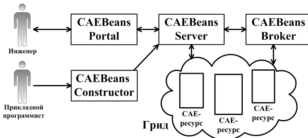
Рис. 3. Общая схема взаимодействия компонентов системы CAEBeans
