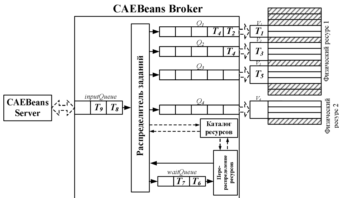
Рис. 5. Структура очередей CAEBeans Broker.
